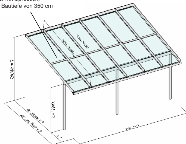
Dachfelder mit Sprossen, geteilt ab Bautiefe von 350 cm
